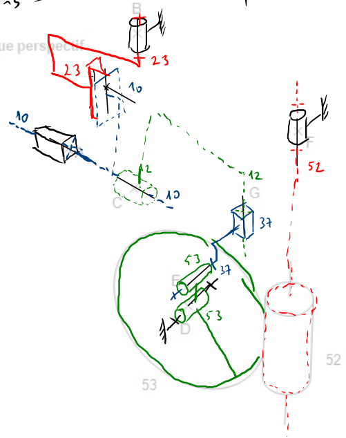
Schéma cinématique perspectif
